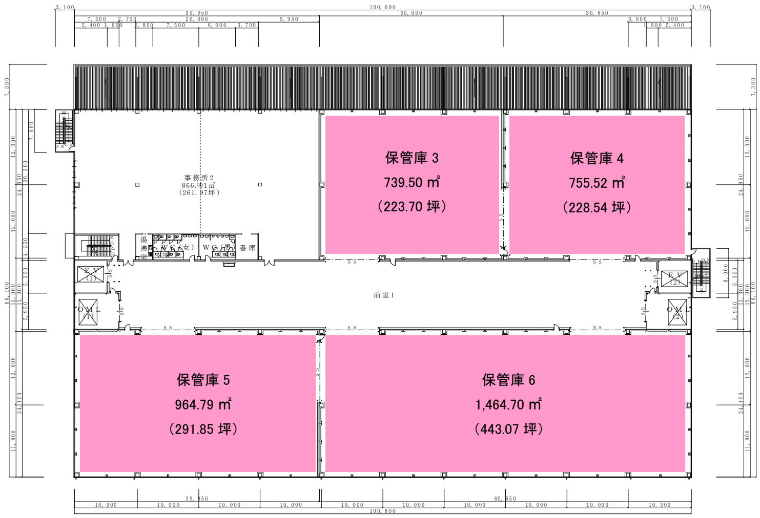
2階平面図 1 / 200
