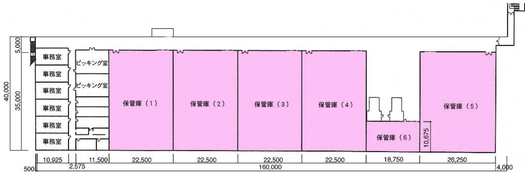
2F平面図
