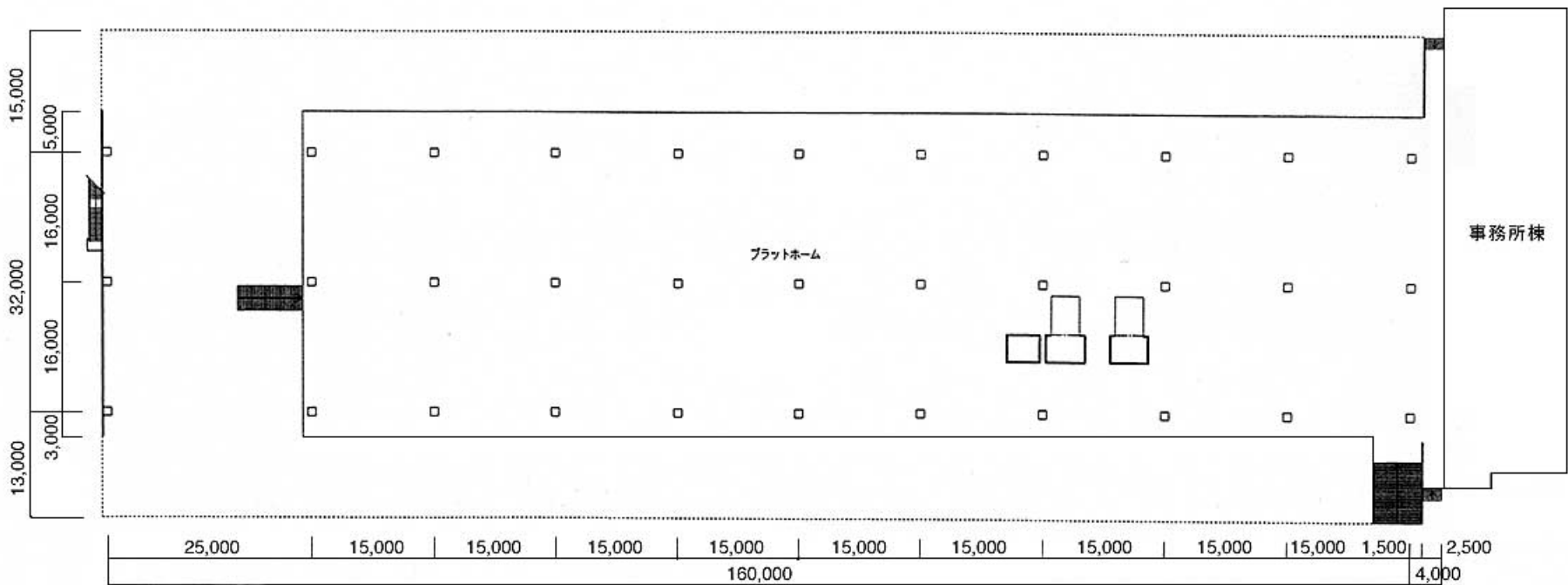
1F平面図
